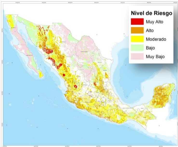
Mapa de riesgo de escarabajos ambrosiales exóticos. Periodo Enero-Marzo
